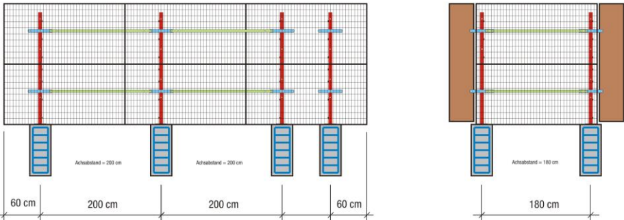
Bild: Querriegel bei Achsabstand 200cm (links) und Achstabstand (180 cm) rechts
