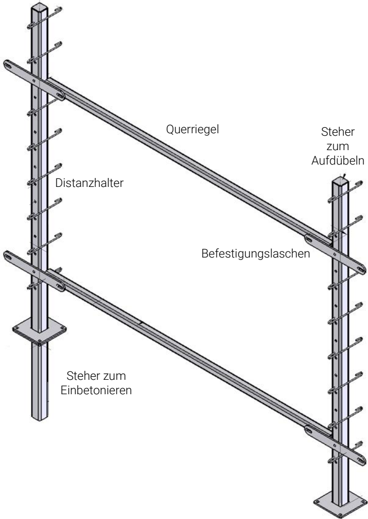
Bild: Aufbau der Zaun-Gabione mit Einzelteilen (Symbolabbildung)
